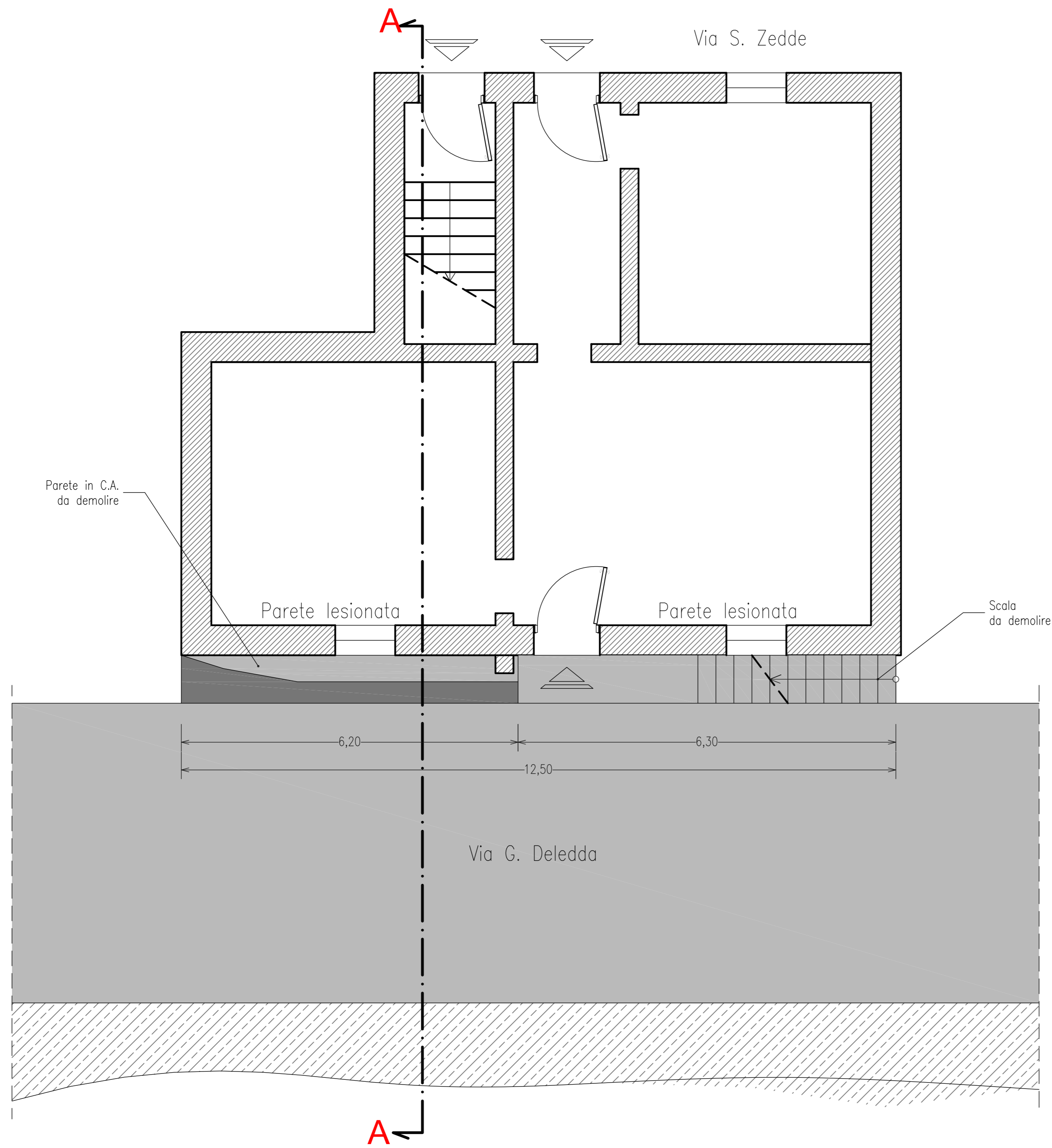
PLANIMETRIA GENERALE ANTE OPERAM (scala 1:50)
